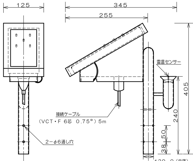
センサー部 GK-72 (縮尺1/7) 材質 受雪板 FRP シャース SUS430 センサー部 塗装色 5Y7/1
