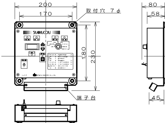
本体制御部 N-21 (縮尺1/7)
