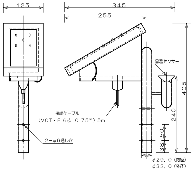
センサー部 GK-71 (縮尺1/7) 材質 受雪板 FRP シャーン SUS430 センサー部 塗装色 5Y7/1
