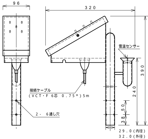
受雪板 G - 5 (縮尺 1/7)
