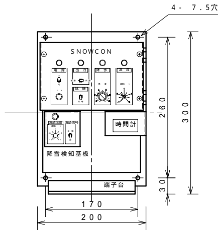
本体 SN - 435 (縮尺 1/7)
