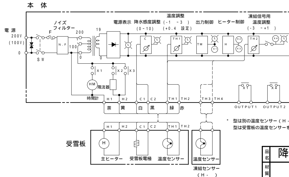
内部接続図
