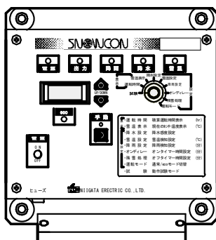
本体制御部
