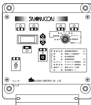
本体制御部
